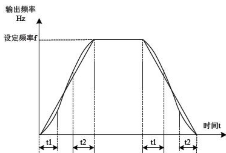
图 7-1-1 变频器的频率特性曲线
